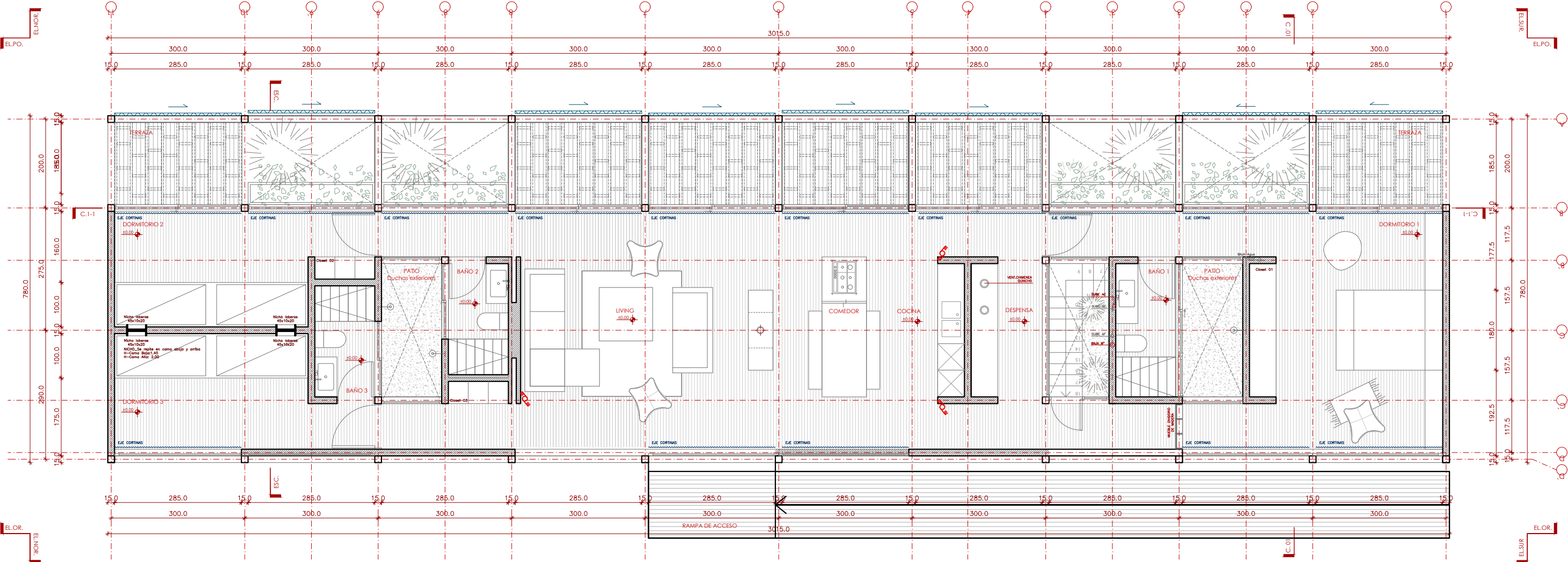
PLANTA ALTA Esc : 1.50
